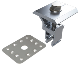
NXT-AU-2 Abrazadera universal p/panel con marco de 25-40 mm
