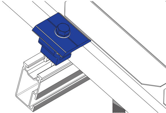
Detalle abrazadera universal, modo abrazadera remate
