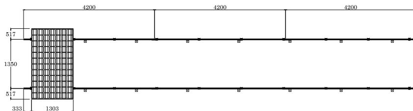
VISTA PLANTA
