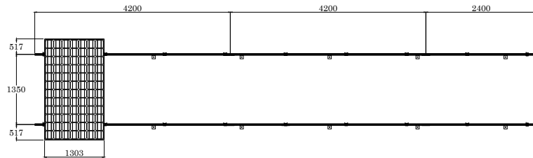
VISTA PLANTA
