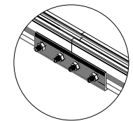
DETALLE D Empalme de Riel
