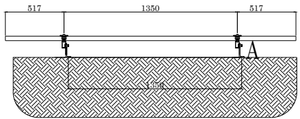
VISTA LATERAL
