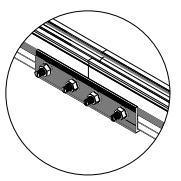
DETALLE D Empalme de Riel
