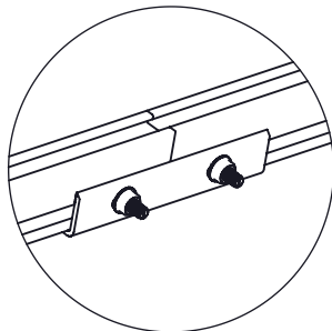
DETALLE "C" NXT-RS Empalme de riel RX
