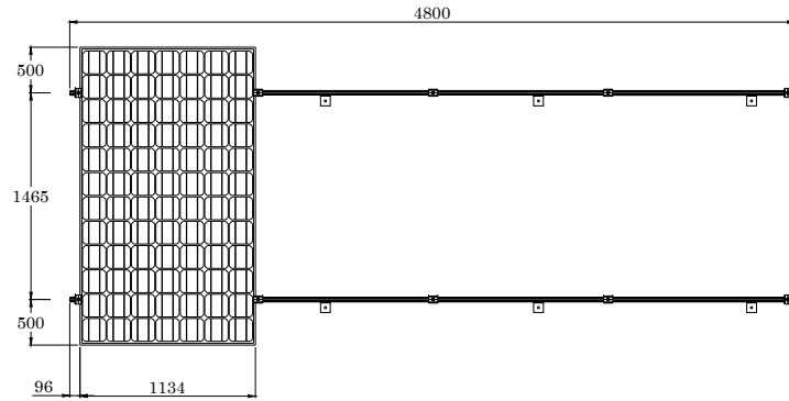
VISTA PLANTA
