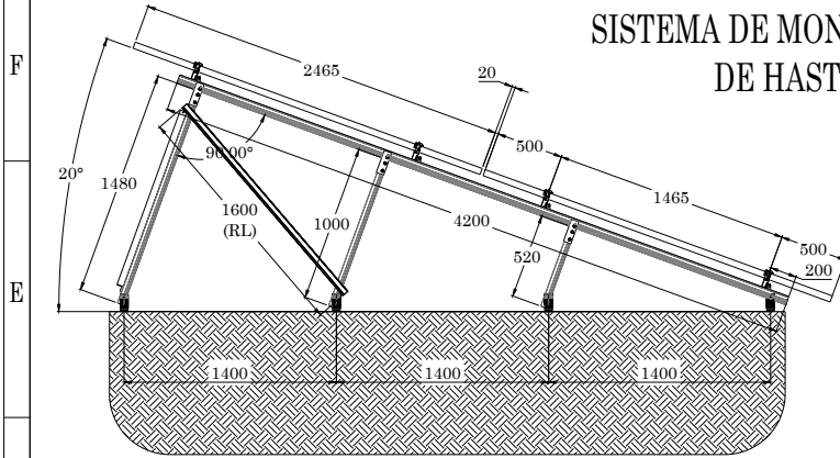
VISTA LATERAL
